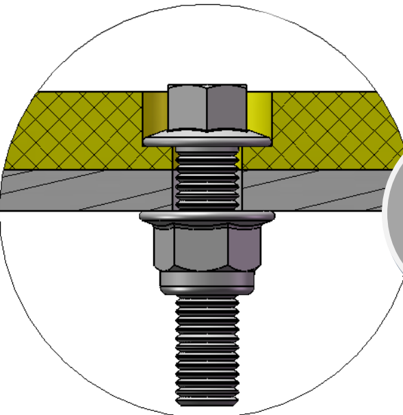
Boulon et écrou
